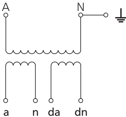
Schaltbildbeispiel einpoliger Spannungswandler mit en-Wicklung
