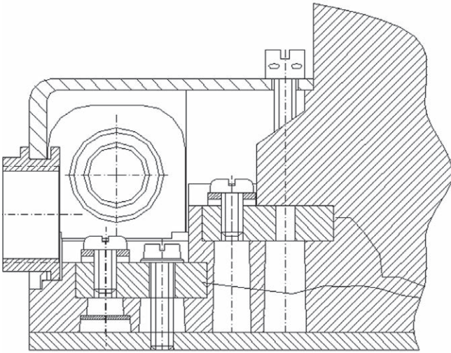
Sekundärbereich mit Erdungsklemme eines Stromwandlers des Typ ASS
