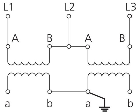
Schaltbildbeispiel V-Schaltung
