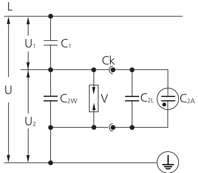
Prinzip-Schaltbild Kapazitiver Spannungsteiler
