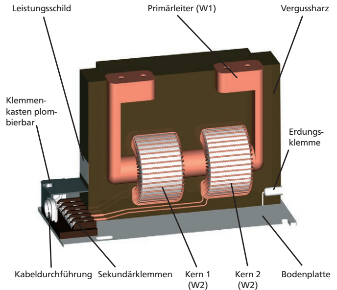
Prinzipielles Schnittbild eines Stromwandlers
