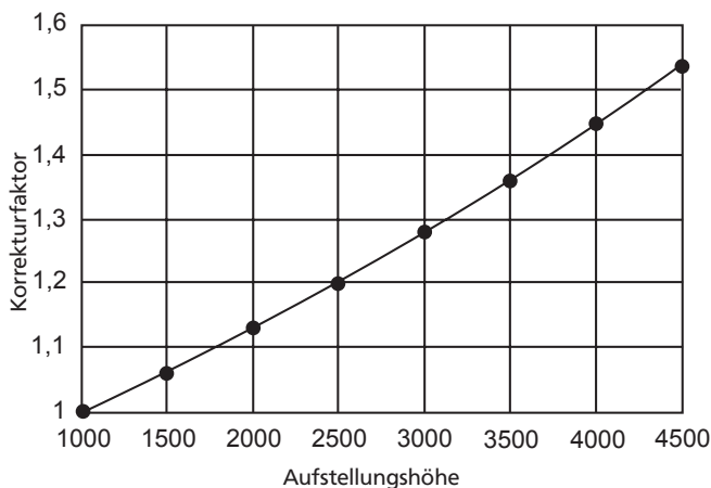
Grafik Höhenkorrekturfaktor
