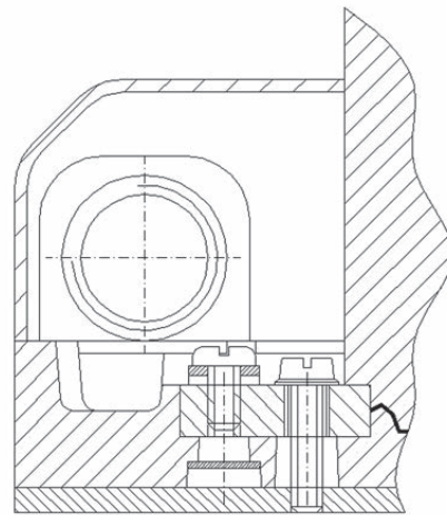
Sekundärbereich mit Erdungsklemme eines Spannungswandlers der Typen VES/VEN
